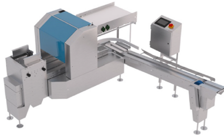
■ FP ONE Estandar – 36.000 Huevos / Hora
