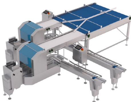
■ Dos FP ONE con Mesa de Distribución – 72.000 Huevos / Hora
